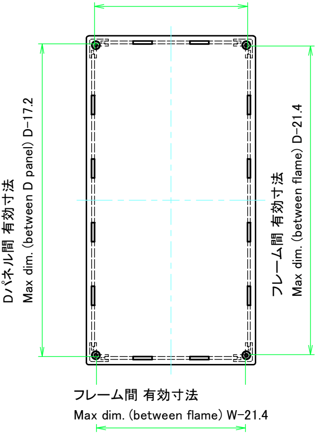
Wパネル間 有効寸法 Max dim. (between W panel) W-17.2
